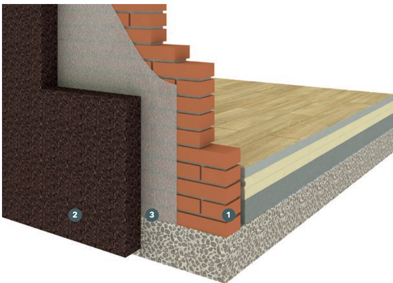
1) Binnenmuur (Mur intérieur) 2) Isolatieplaten speciaal facade (Panneaux d'isolation spécial façade) 3) Lijmlaag (Couche de colle)
